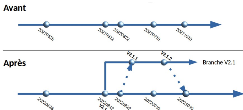
Figure 3: Gestion de versions via des branches de code.
